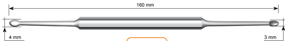
Ложка кюретажная №1 110-001 Bone curette №1
