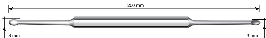
Ложка кюретажная №3 110-003 Bone curette №3
